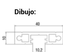
Perfil de Aluminio
